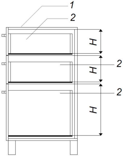
Figura 13.1: Altura livre
